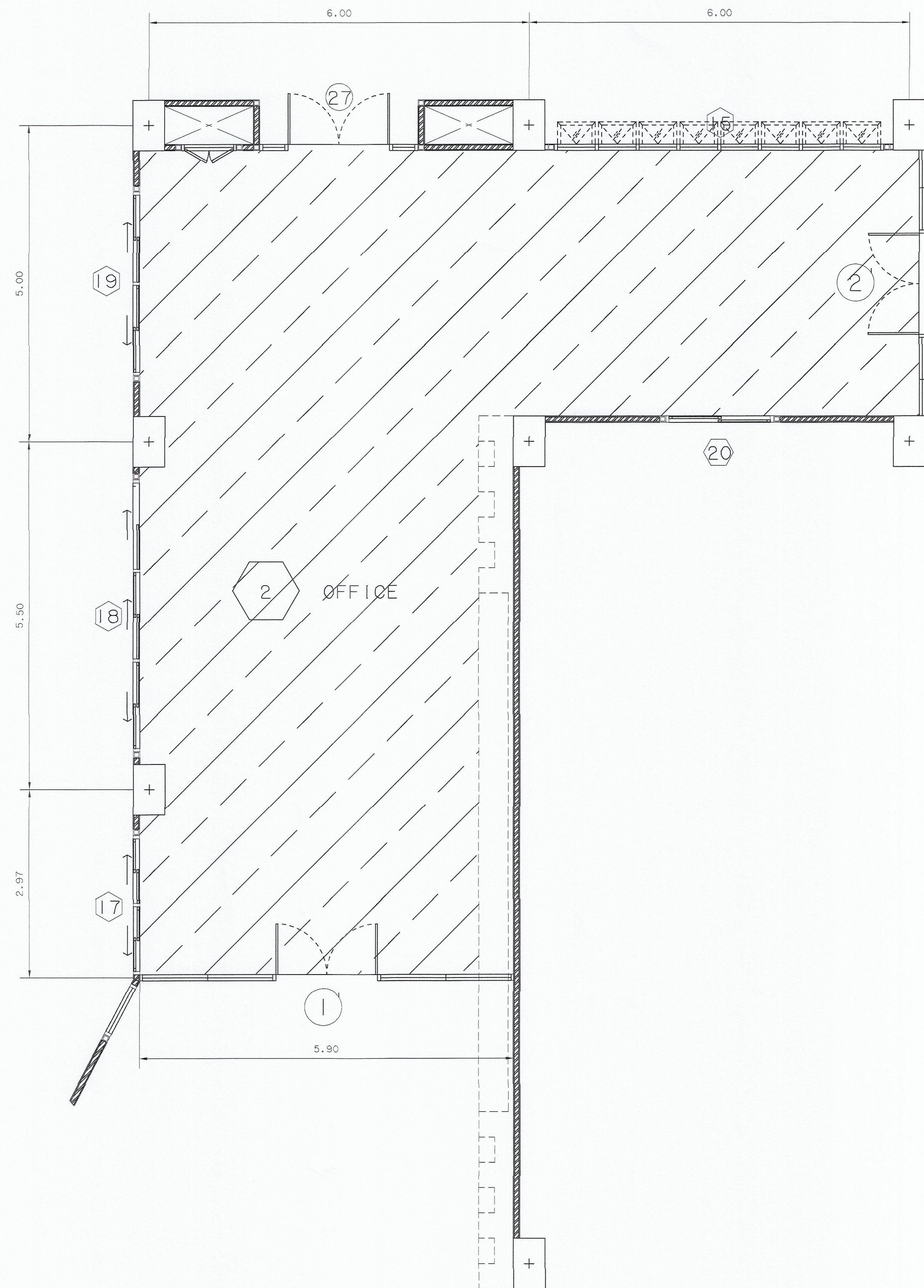
แปลน OFFICE มาตราส่วน 1:50
