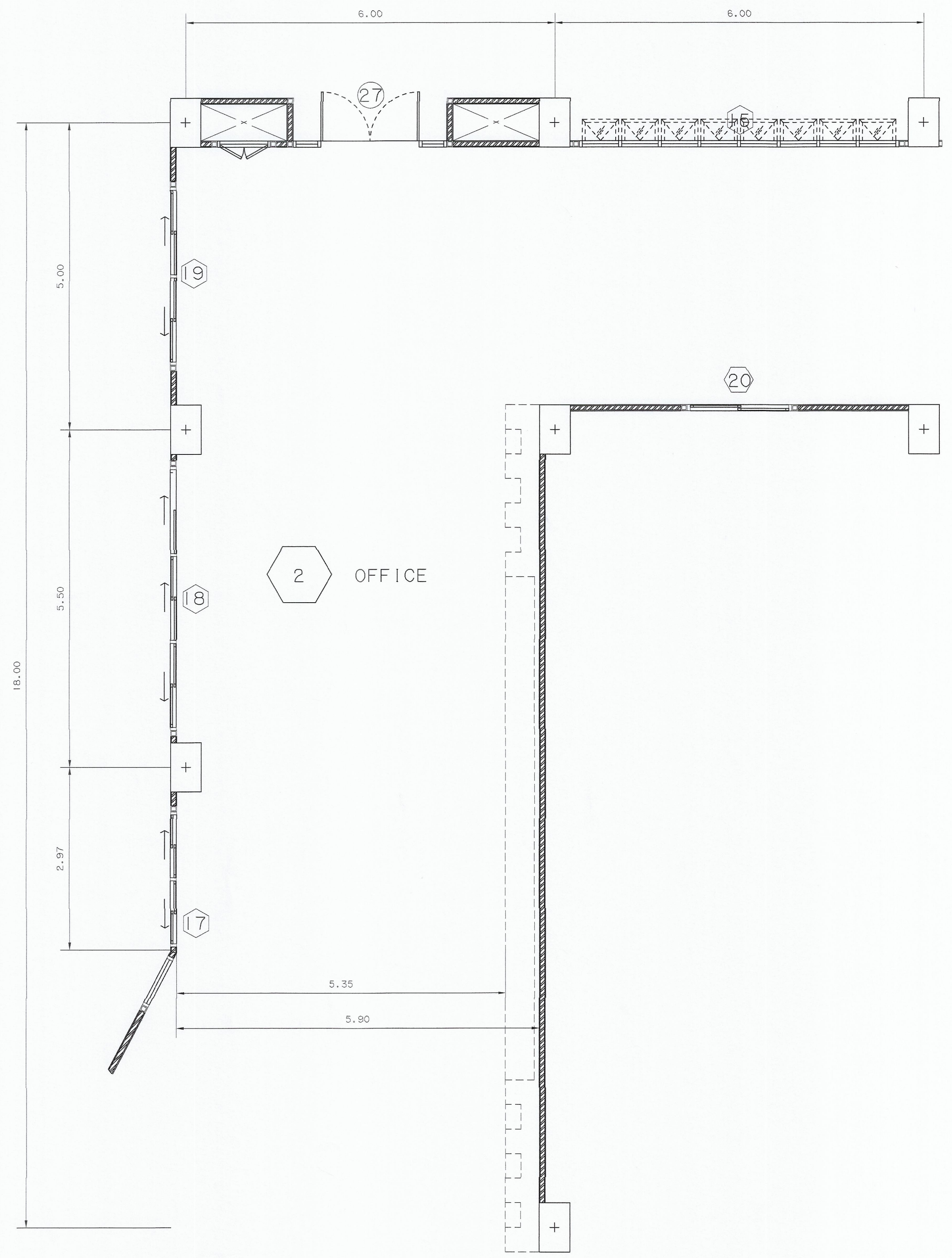
แปลน OFFICE มาตรฐาน 1 : 50 ก่อนการปรับปรุง
