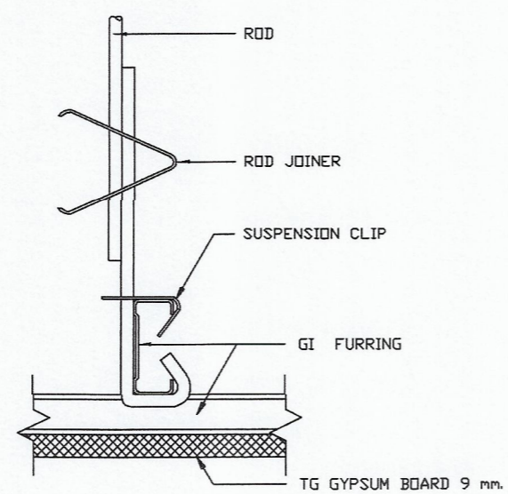
SECTION A SCALE 1 : 2
