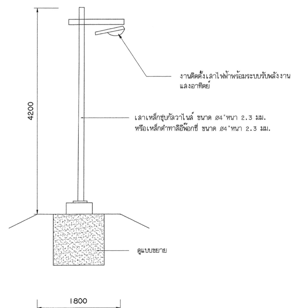
แบบติดตั้งเสาไฟฟ้า N. T. S
