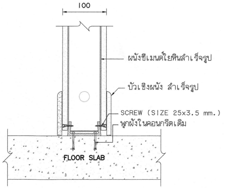
แบบขยายติดตั้งบัวสำเร็จรูป N.T.S กรณีติดตั้งบัวใหม่ (ติดตั้ง2ด้าน)
