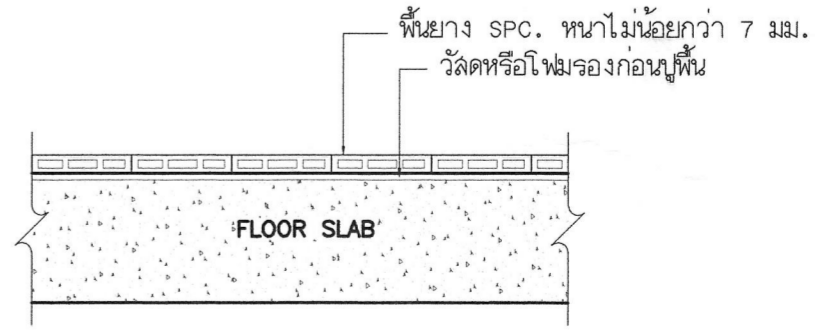
แบบขยายติดตั้งพื้นสำเร็จรูป N.T.S
