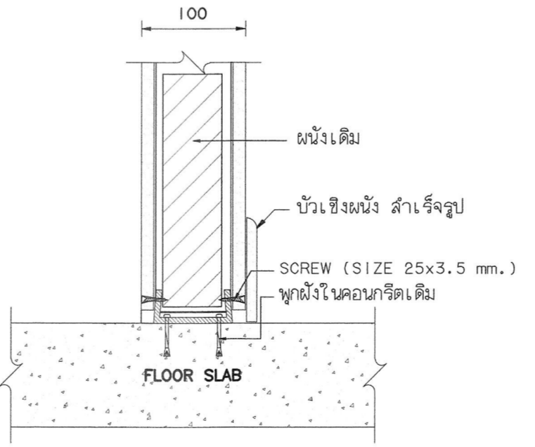
แบบขยายติดตั้งบัวสำเร็จรูป N.T.S กรณีติดตั้งบัวเดิม
