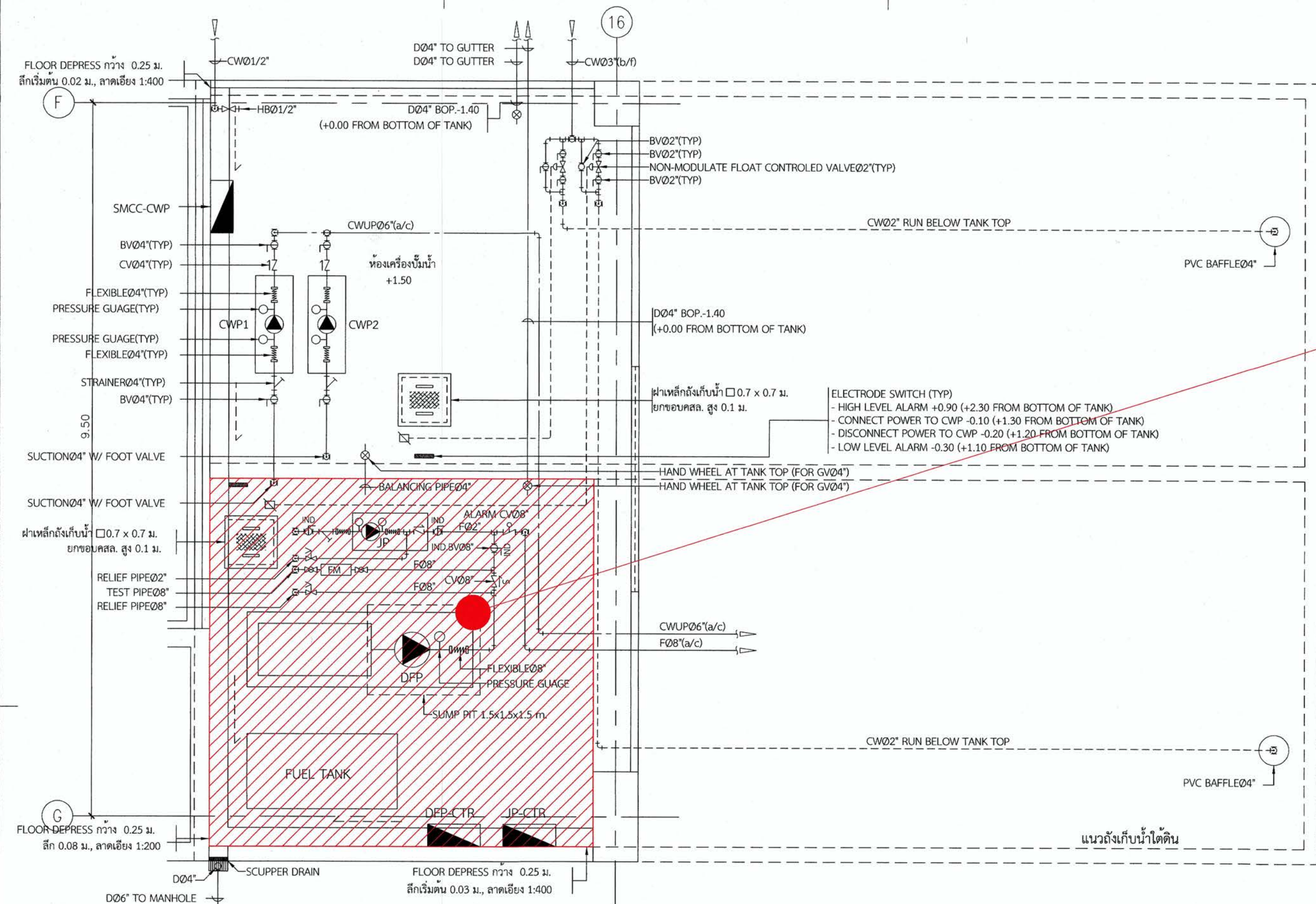
แบบขยายของเครื่องชั้นที่ 1 มาตรฐาน 1:50
