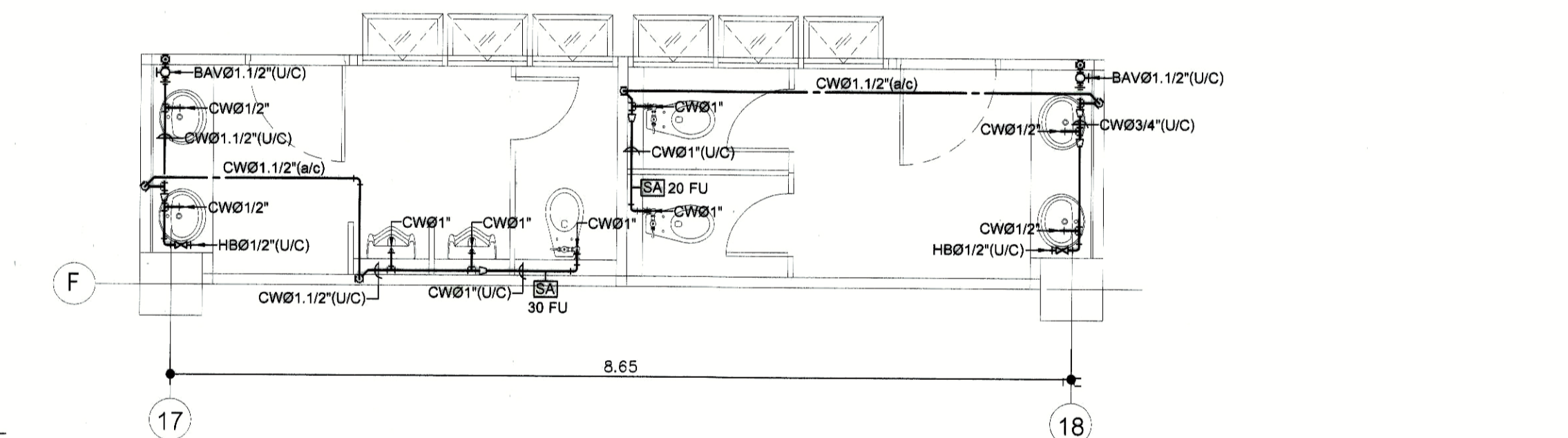
ห้องน้ำ T-103, T-104 (CW) มาตรฐาน 1:50
