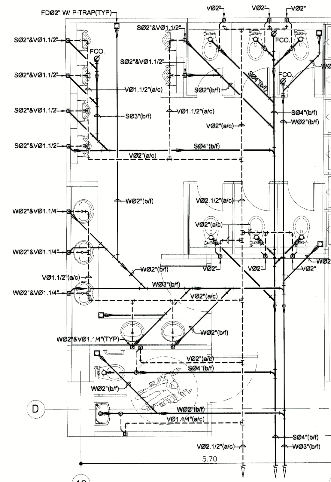
ห้องน้ำ T-502, T-503 (S,W,V) มาตรฐาน 1:50
