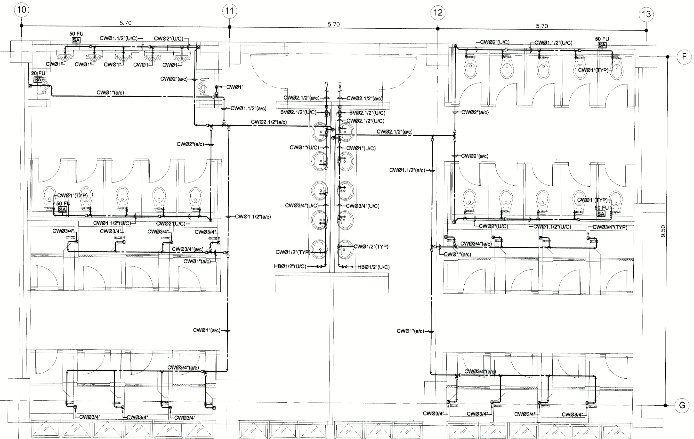
ห้องน้ำ T-204, T-205 (CW) มาตรฐาน 1:50
