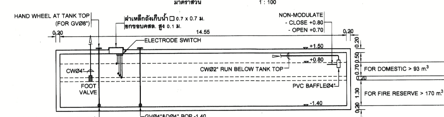
รูปตัด 1-1 มาตราส่วน 1:100
