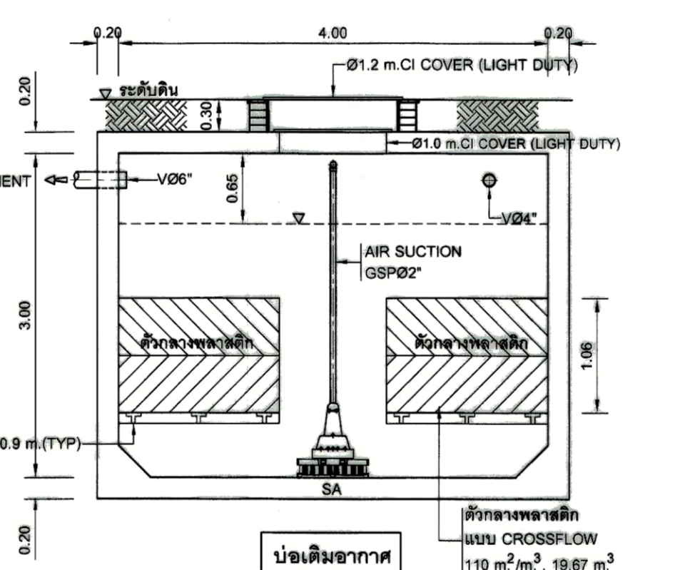
รูปตัด 5-5 มาตราส่วน 1:50
