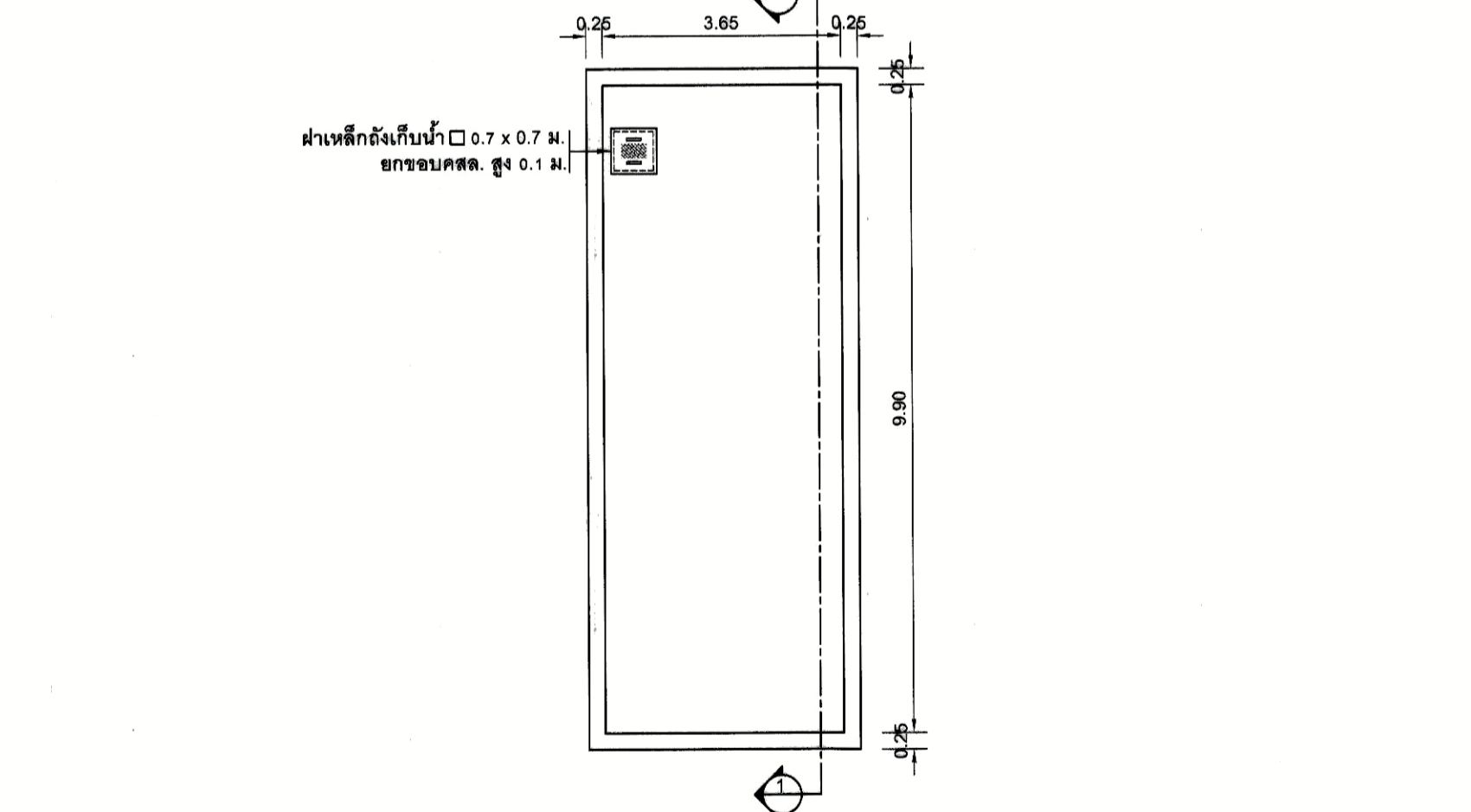
แปลนถังเก็บน้ำควดฟ้า รูปตัด 1-1 มาตราส่วน 1:100
