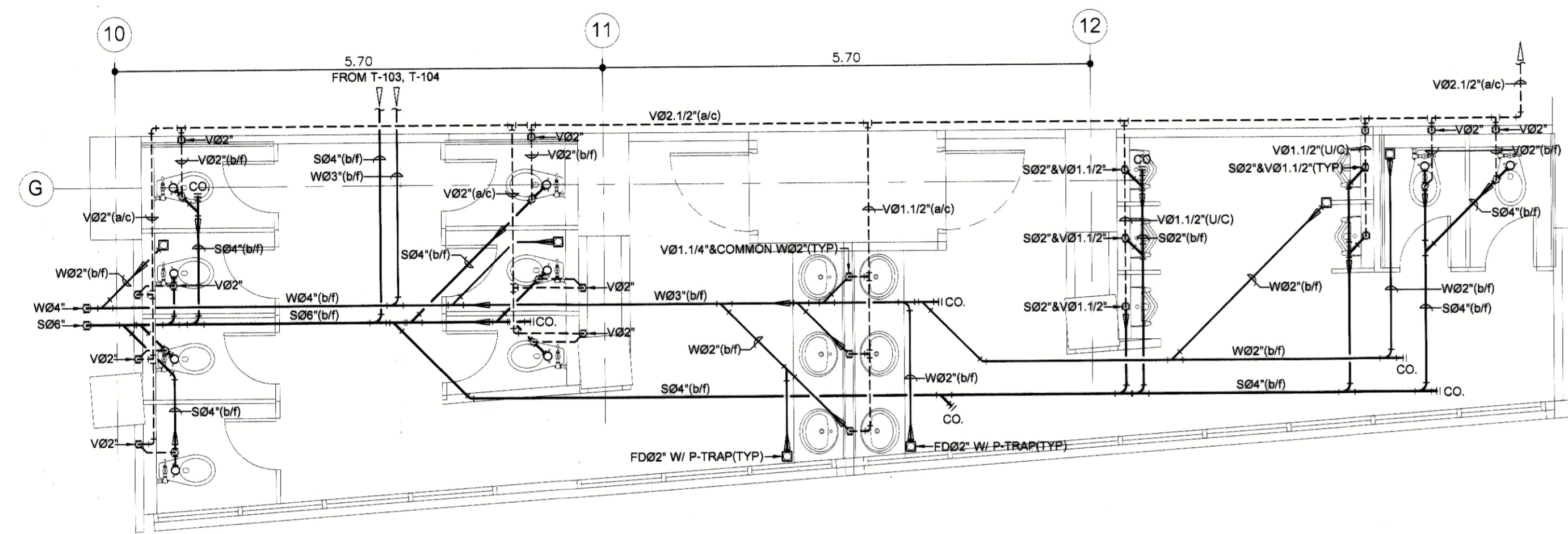
ห้องน้ำ T-101, T-102 (CW) มาตราส่วน 1:50
