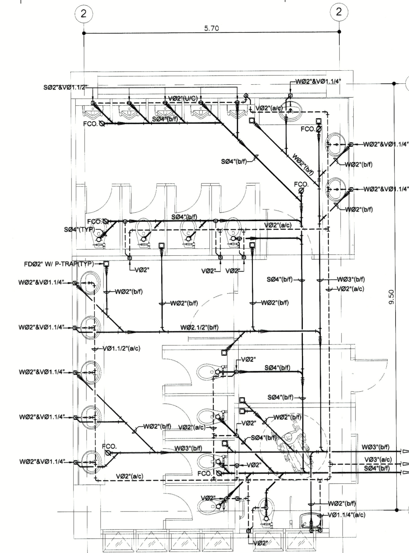
ห้องน้ำ T-201, T-202, T-203 (CW) มาตราส่วน 1:50
