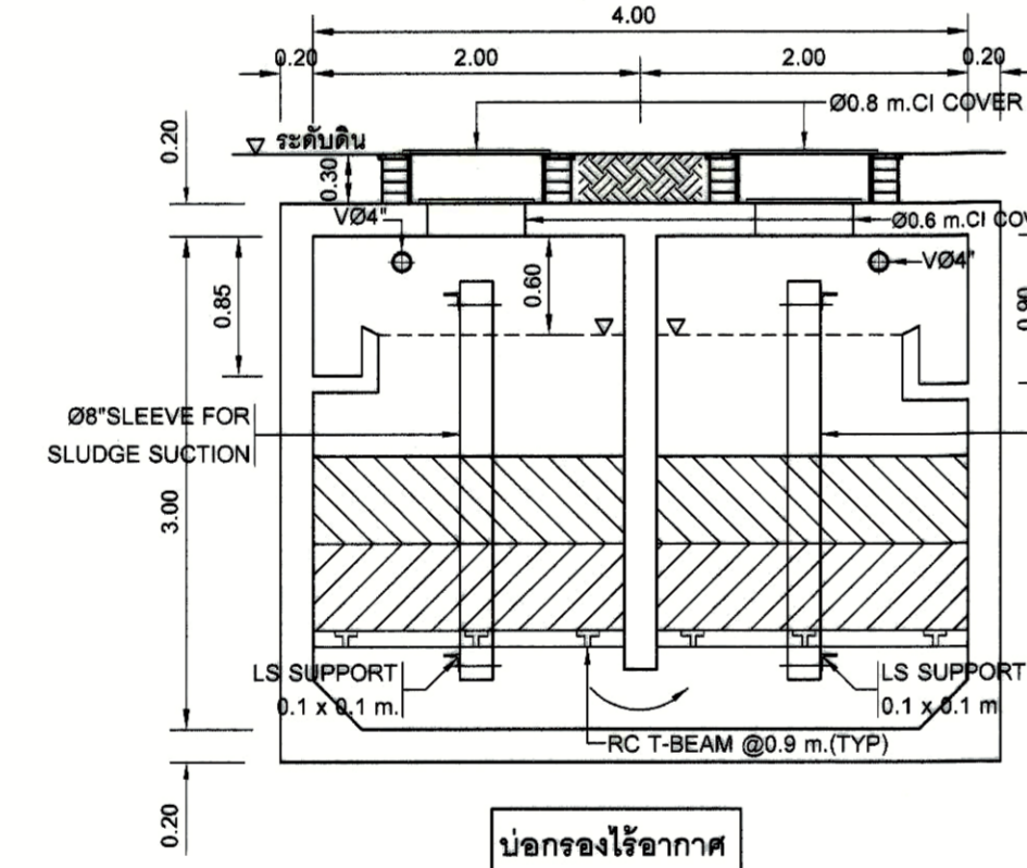
รูปตัด 4-4 มาตราส่วน 1:50
