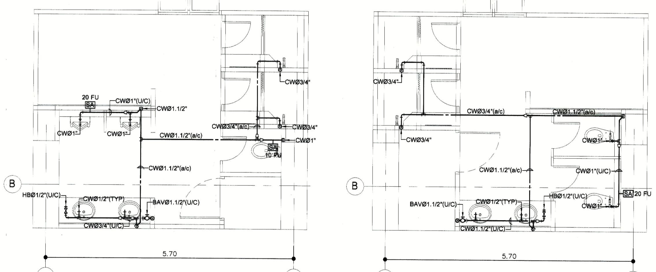
ห้องน้ำ T-105 (CW) มาตรฐาน 1:50
