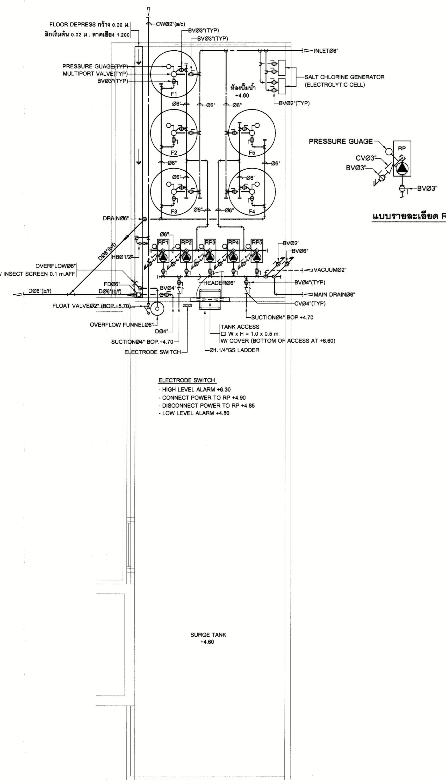
แบบขยายห้องเครื่องสระว่ายน้ำ มาตรฐาน 1:50
