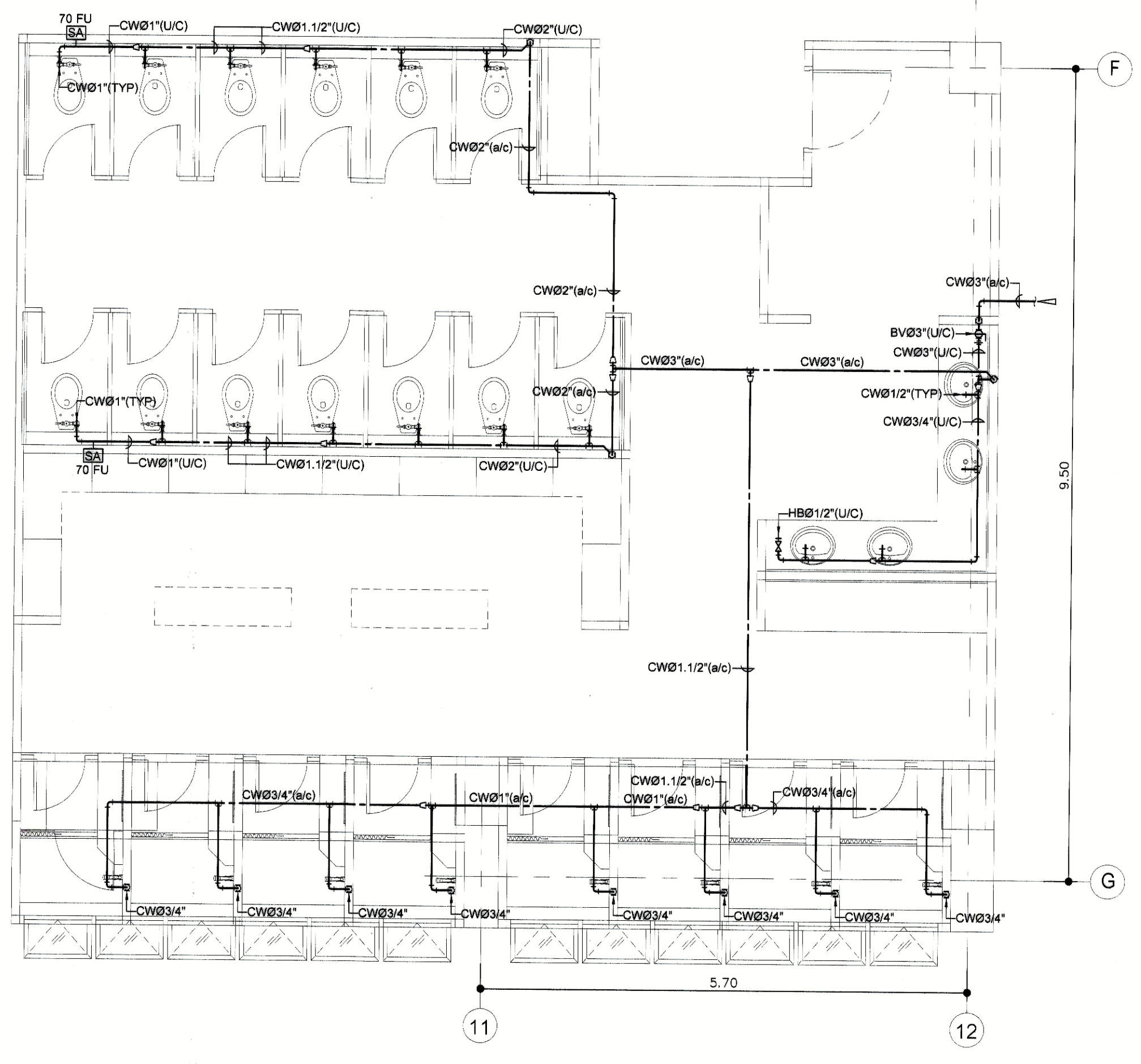
ห้องน้ำ T-401 (CW) มาตราส่วน 1:50
