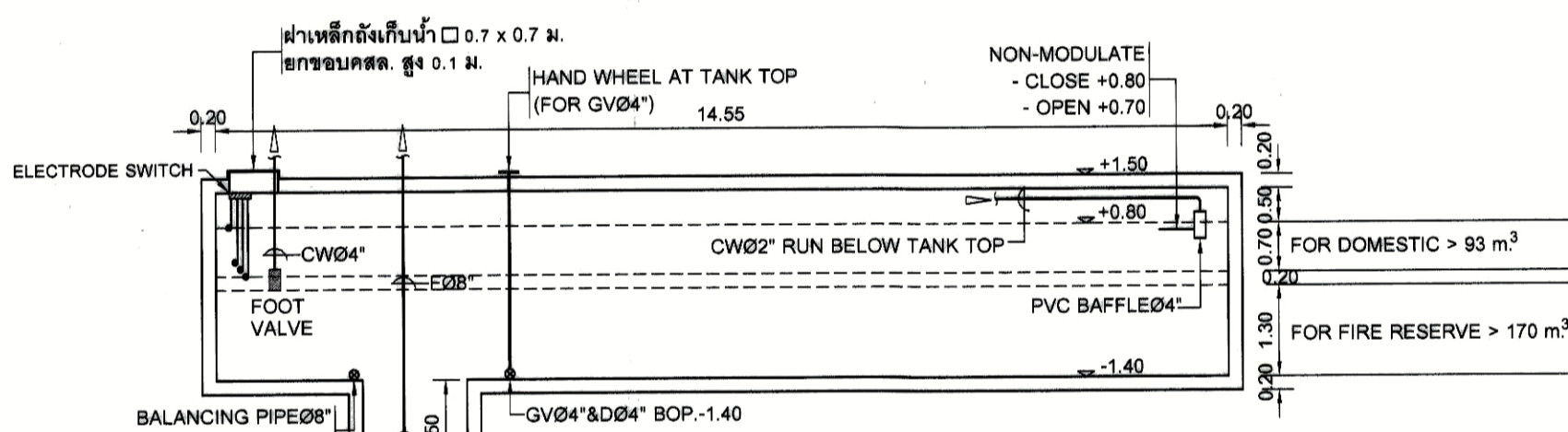
รูปตัด 2-2 มาตราส่วน 1:100
