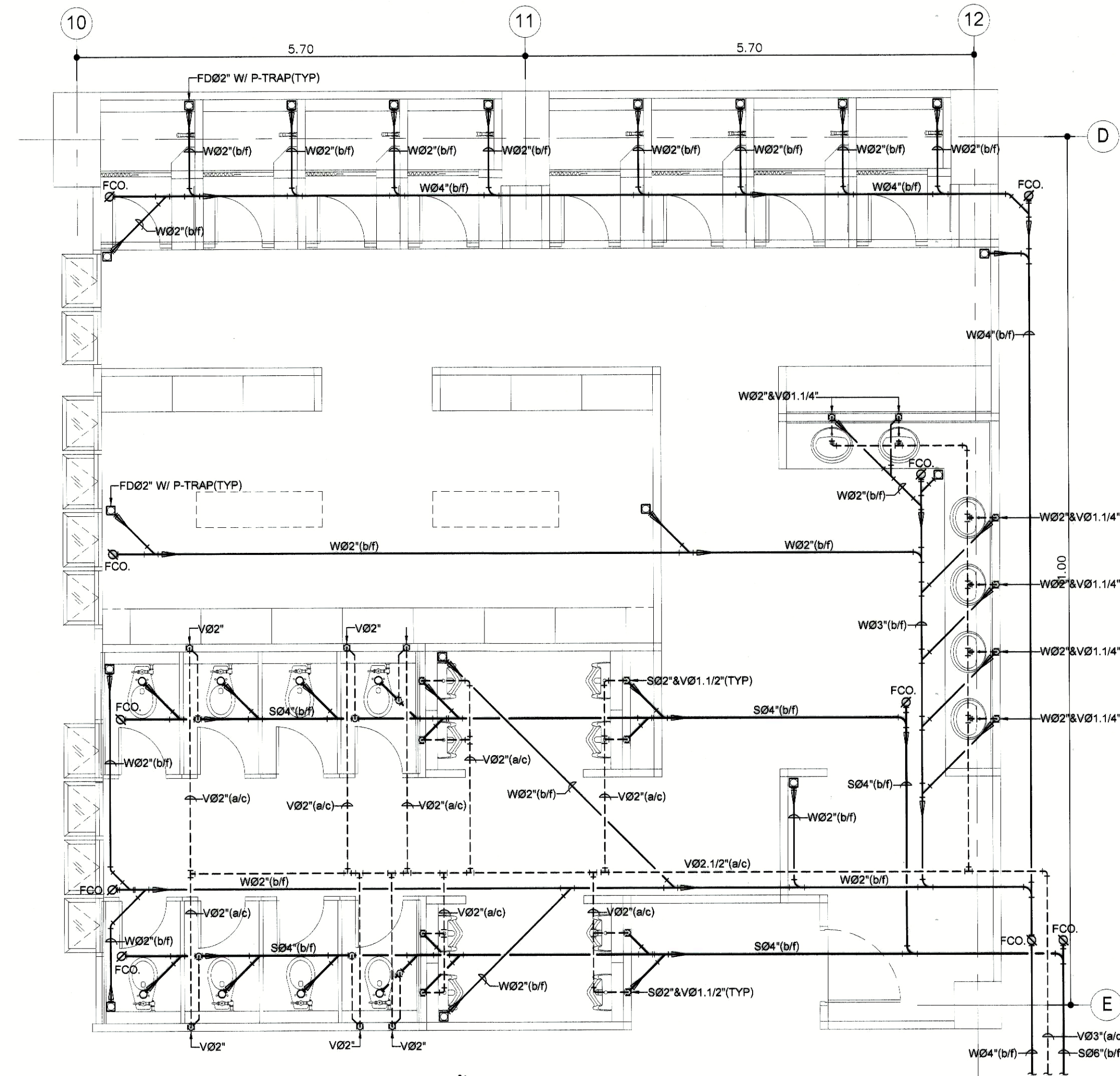
ห้องน้ำ T-402 (CW) มาตรฐาน 1:50
