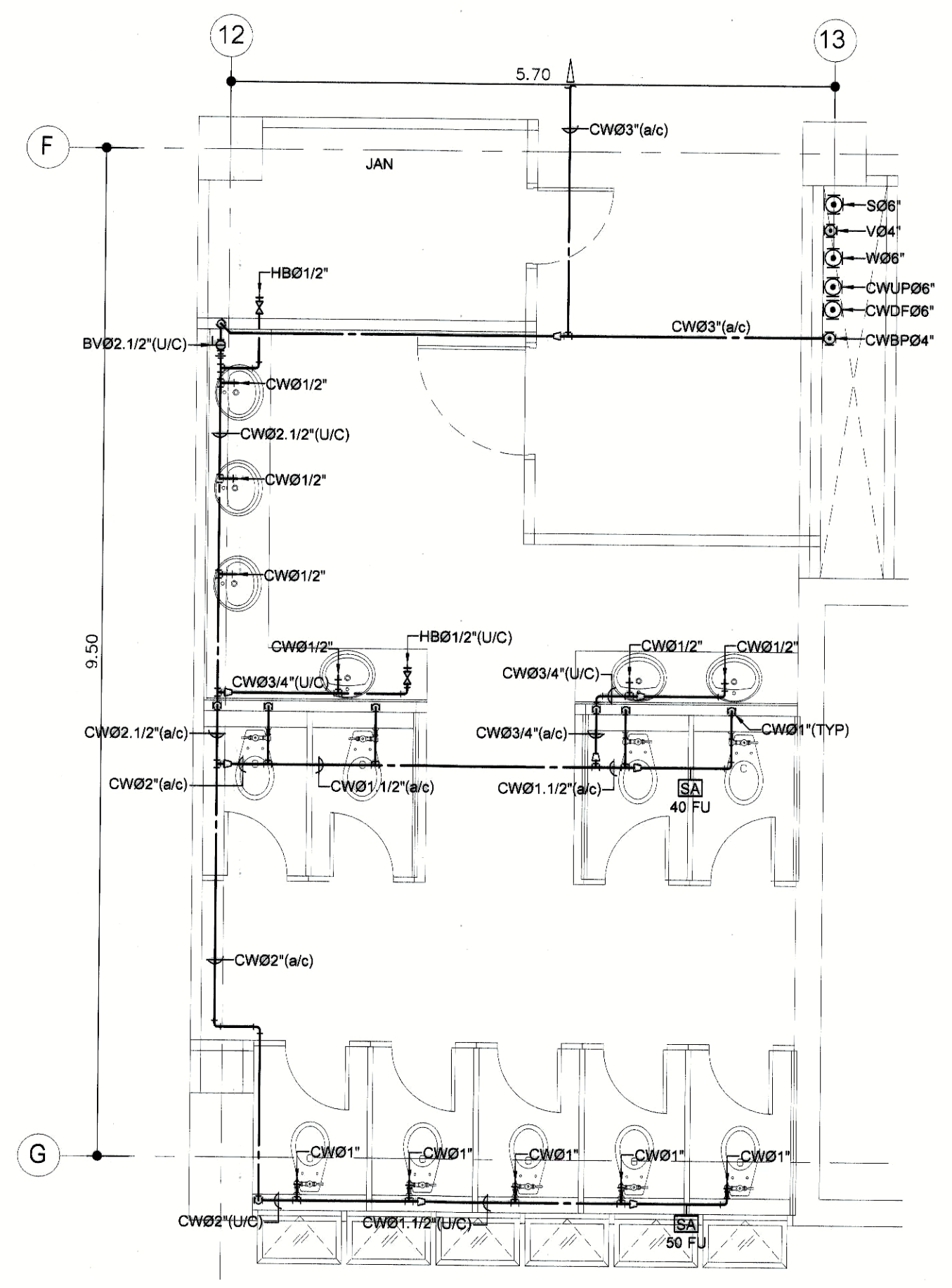
ห้องน้ำ T-501 (CW) มาตราส่วน 1:50
