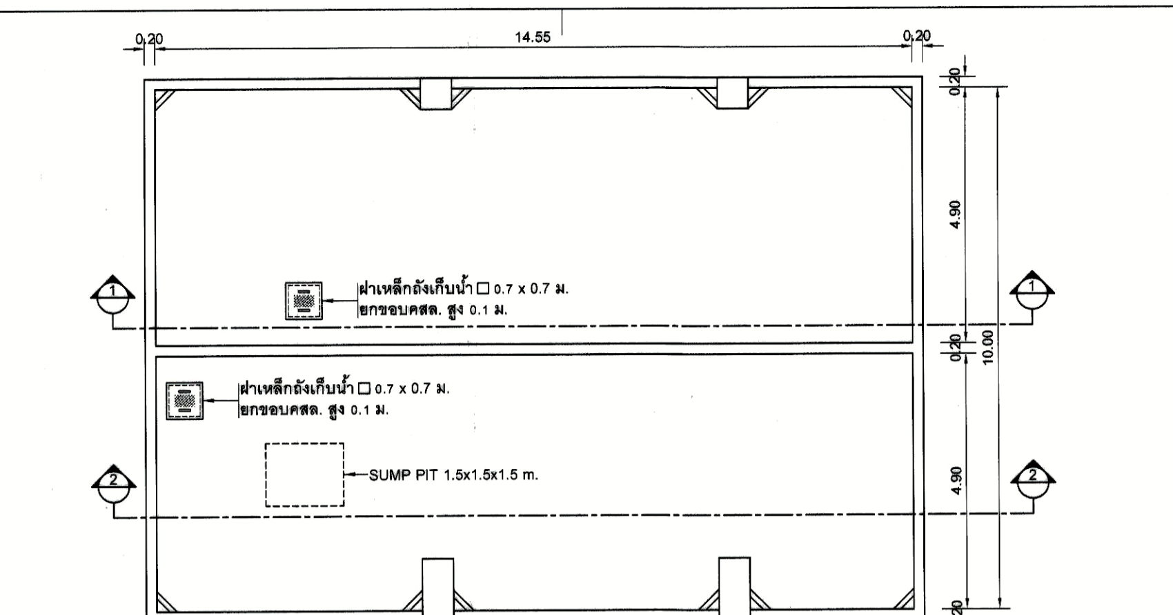
แปลนถังเก็บน้ำใต้ดิน รูปตัด 1-1 มาตราส่วน 1:100
