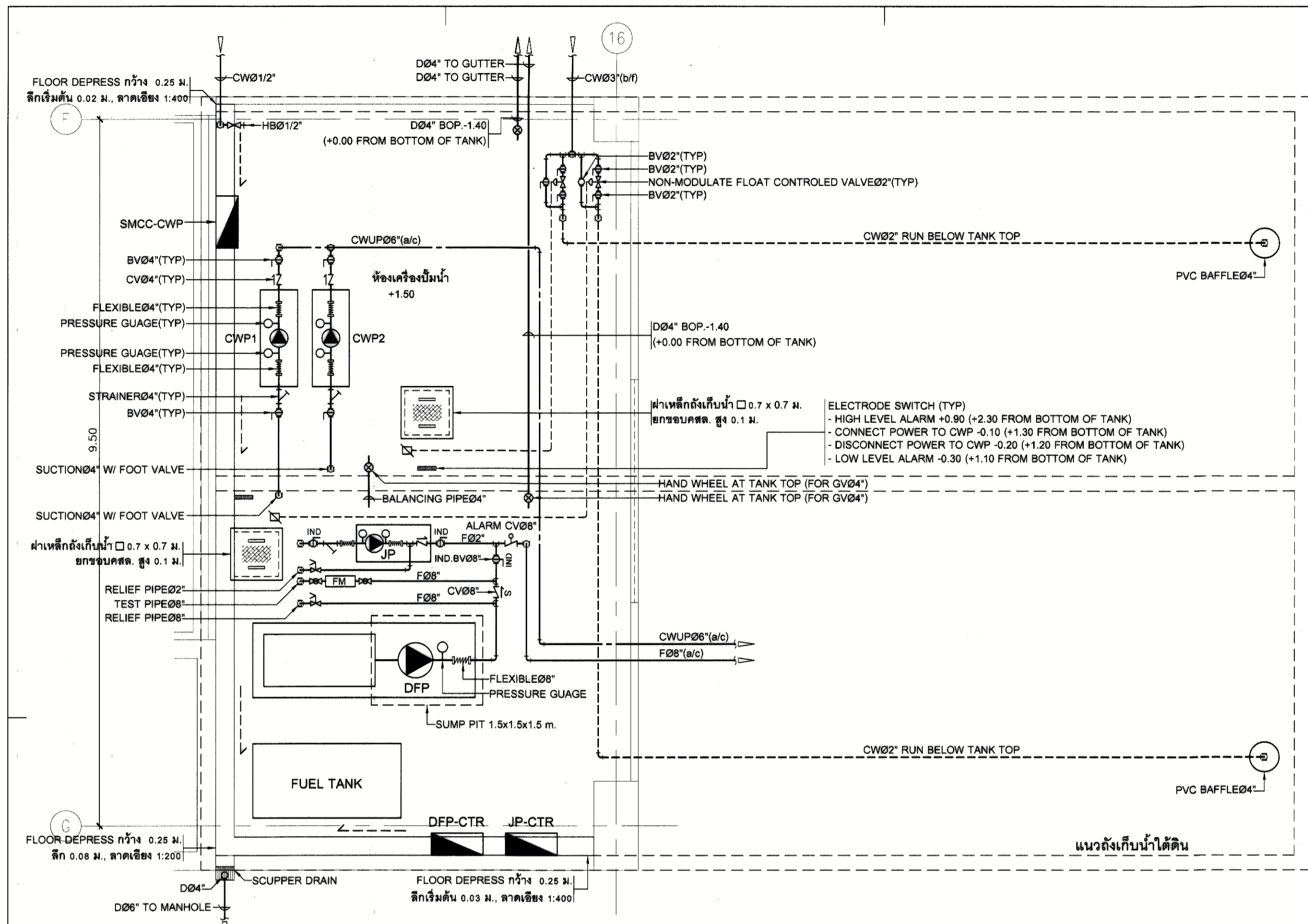
แบบขยายห้องเครื่องชั้นที่ 1 มาตราส่วน 1:50
