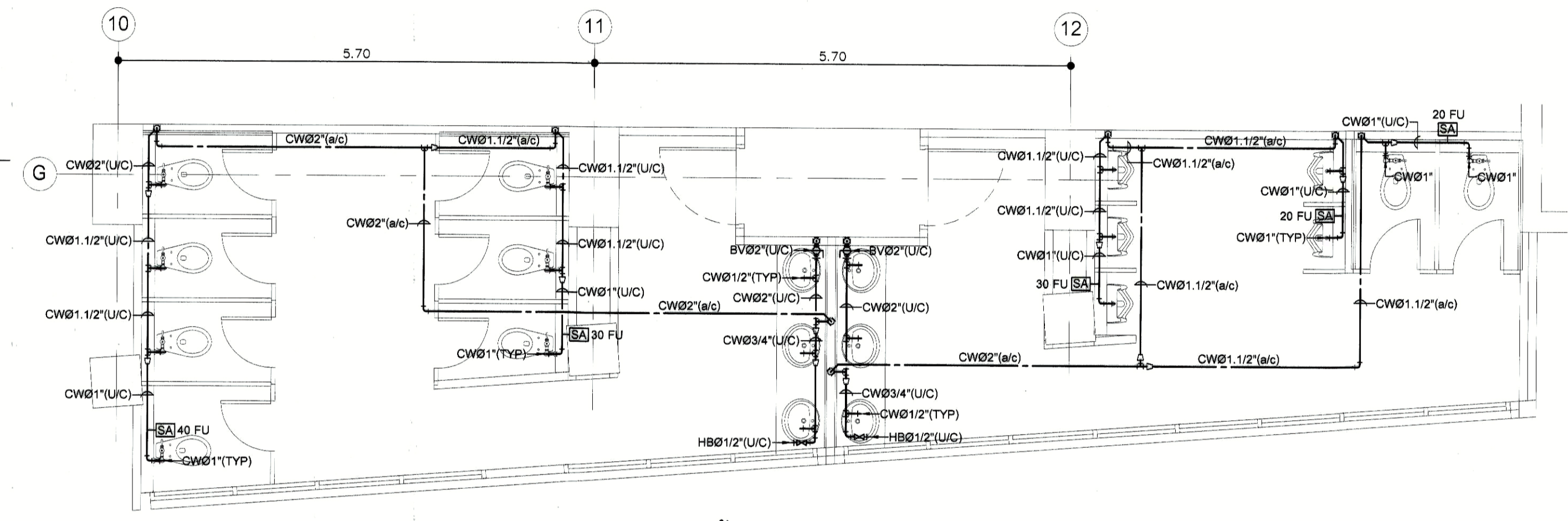
ห้องน้ำ T-101, T-102 (CW) มาตรฐาน 1:50
