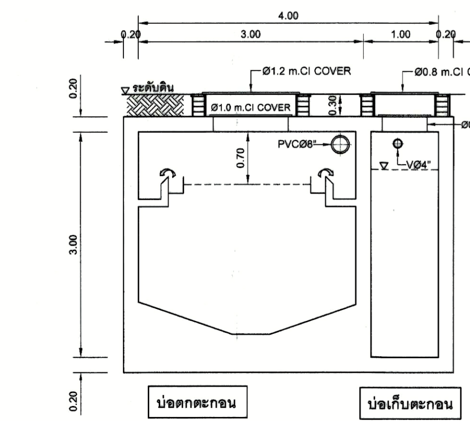
รูปตัด 6-6 มาตราส่วน 1:50
