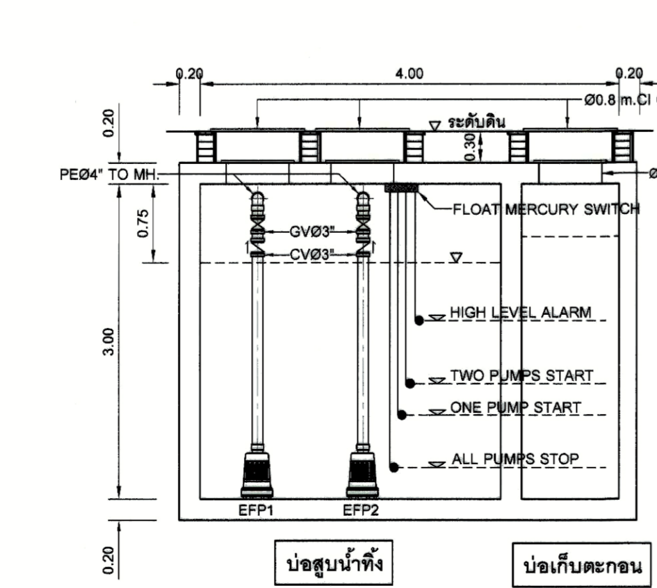
รูปตัด 7-7 มาตราส่วน 1:50
