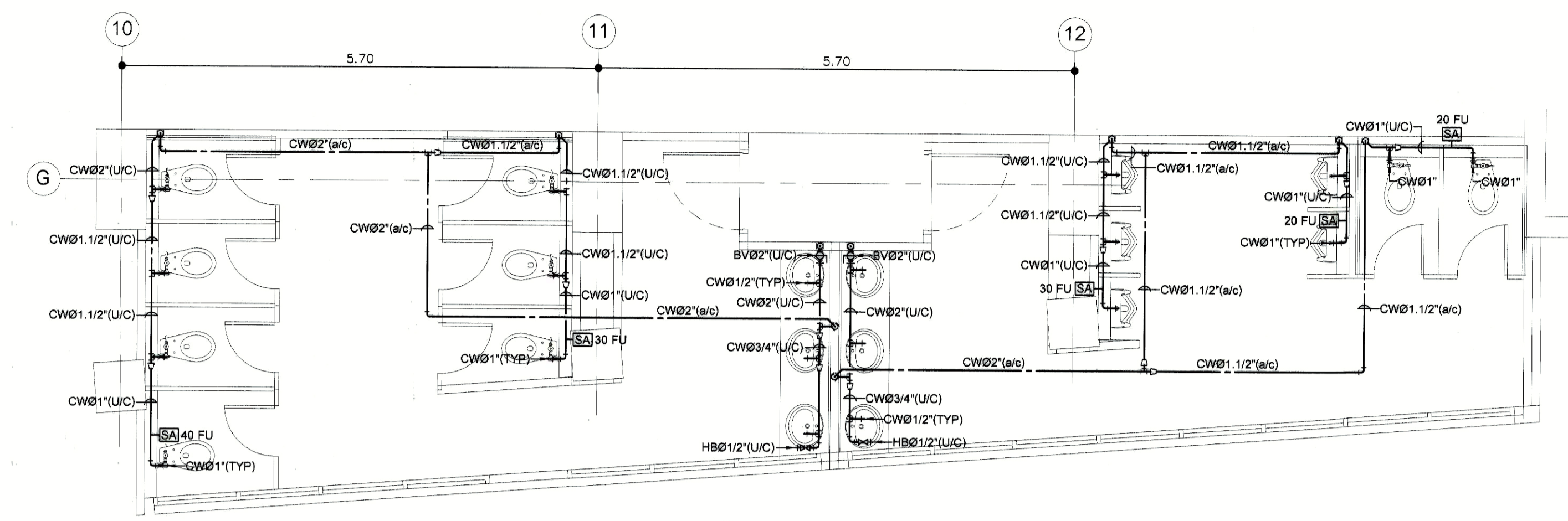
ห้องน้ำ T-G01, T-G02 (CW) มาตรฐาน 1:50
