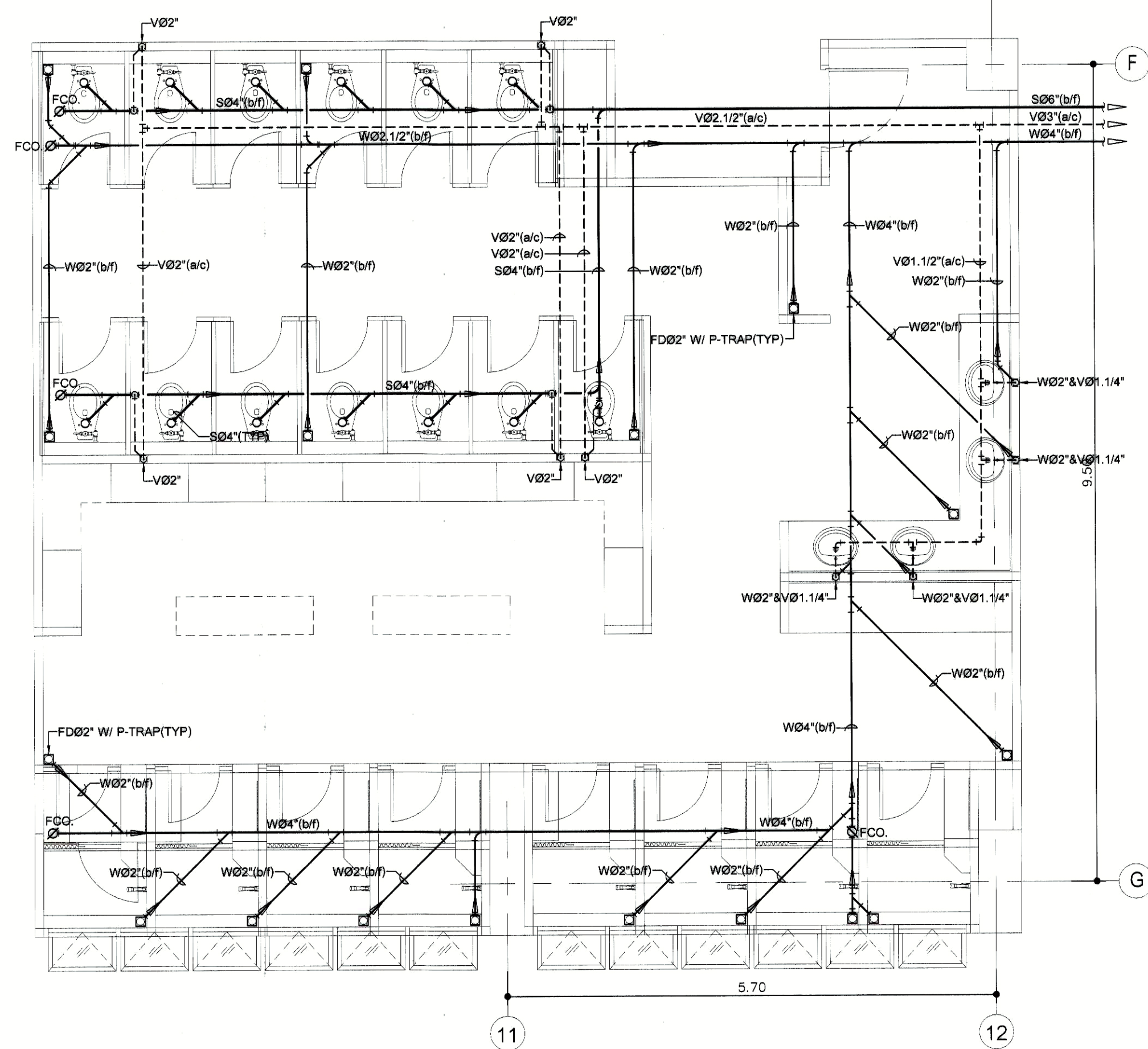
ห้องน้ำ T-401 (CW) มาตรฐาน 1:50
