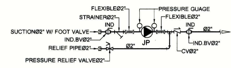
แบบการติดตั้งปั๊ม JP
