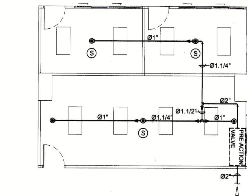
แบบระบบ PRE-ACTION ห้องควบคุม มาตราส่วน 1 : 100
