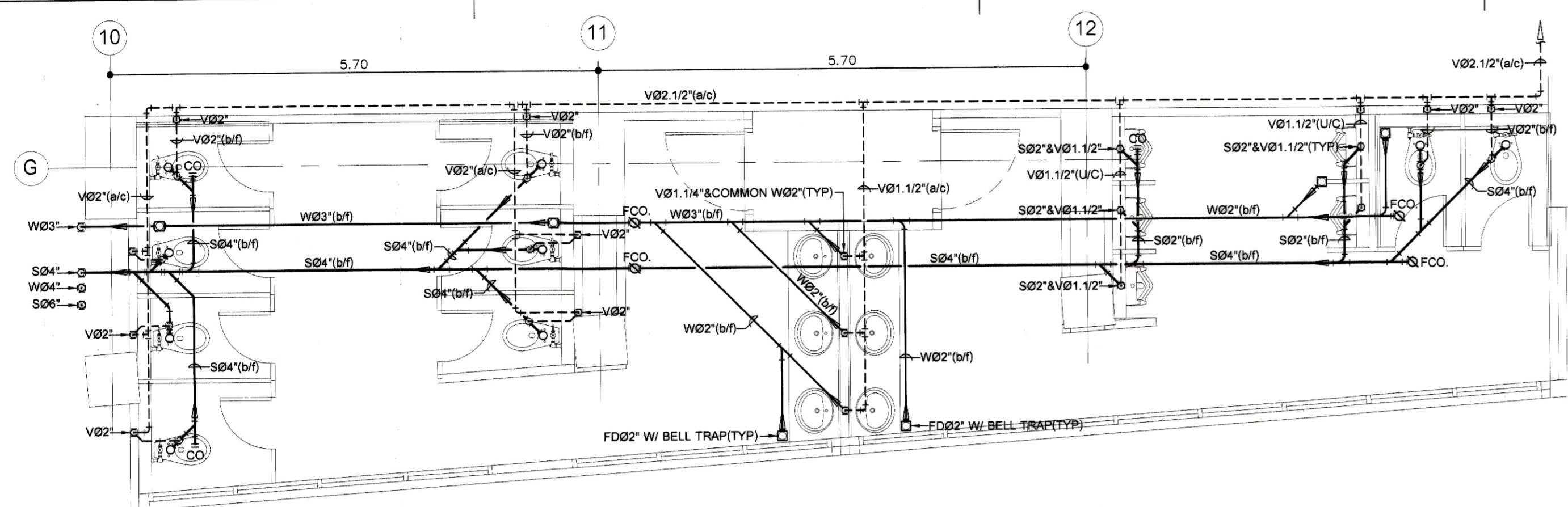
ห้องน้ำ T-G01, T-G02 (CW) มาตราส่วน 1:50
