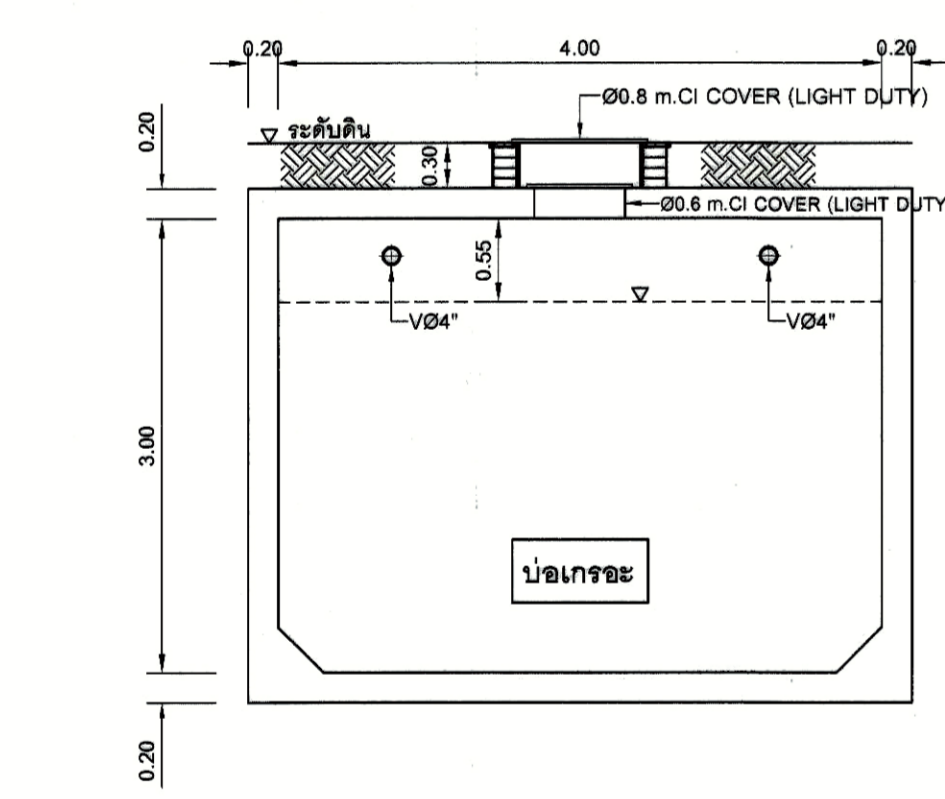
รูปตัด 3-3 มาตราส่วน 1:50
