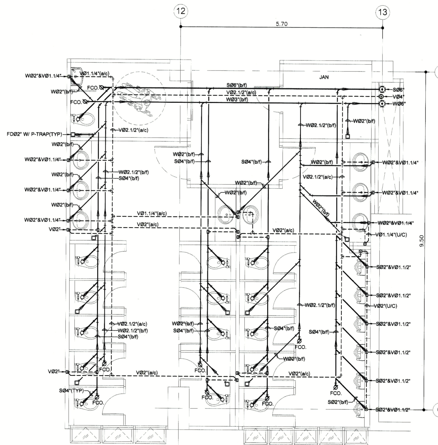
ห้องน้ำ T-301, T-302, T-303 (CW)
