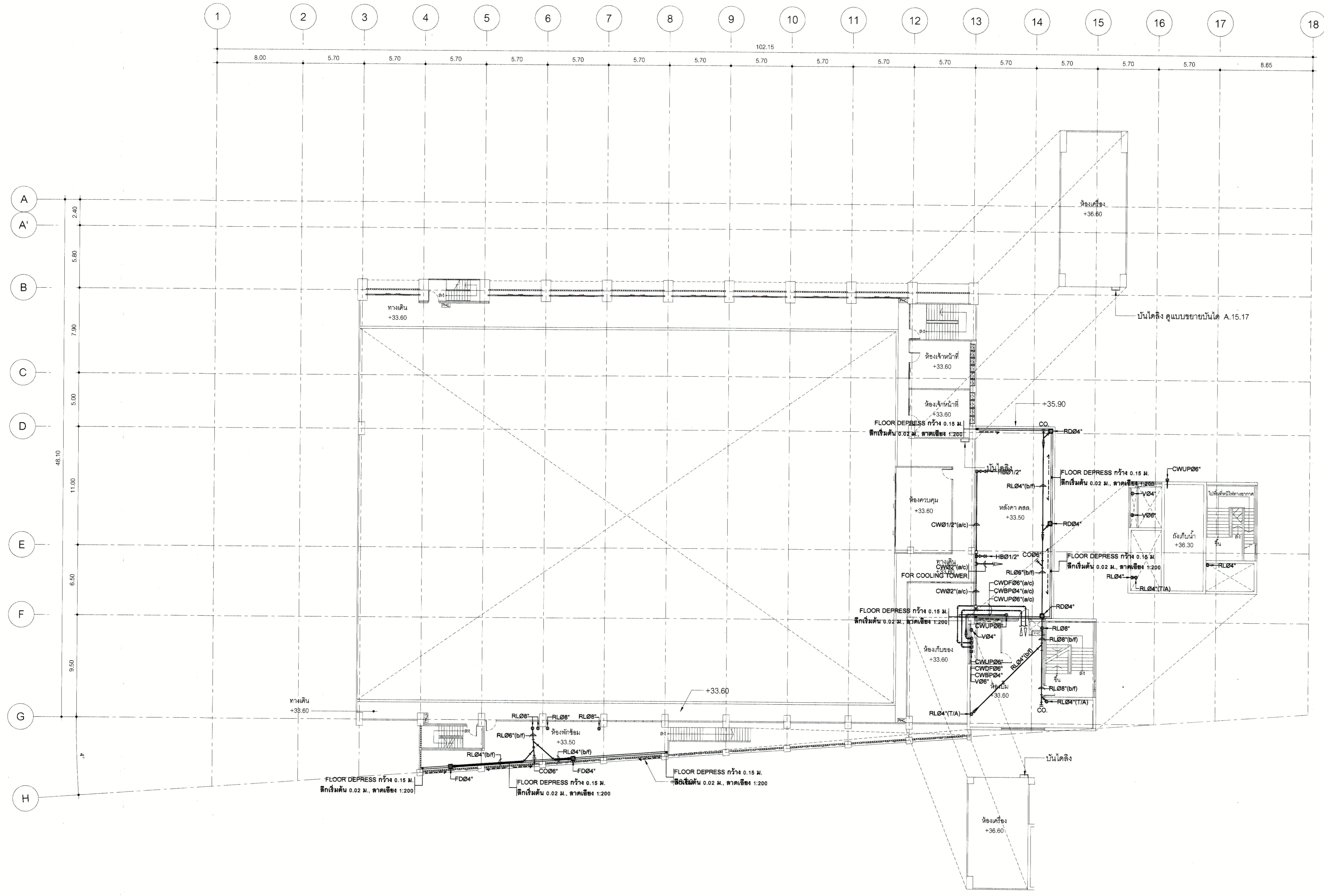
ผังระบบสุขาภิบาลชั้นลอย มาตราส่วน 1: 200
