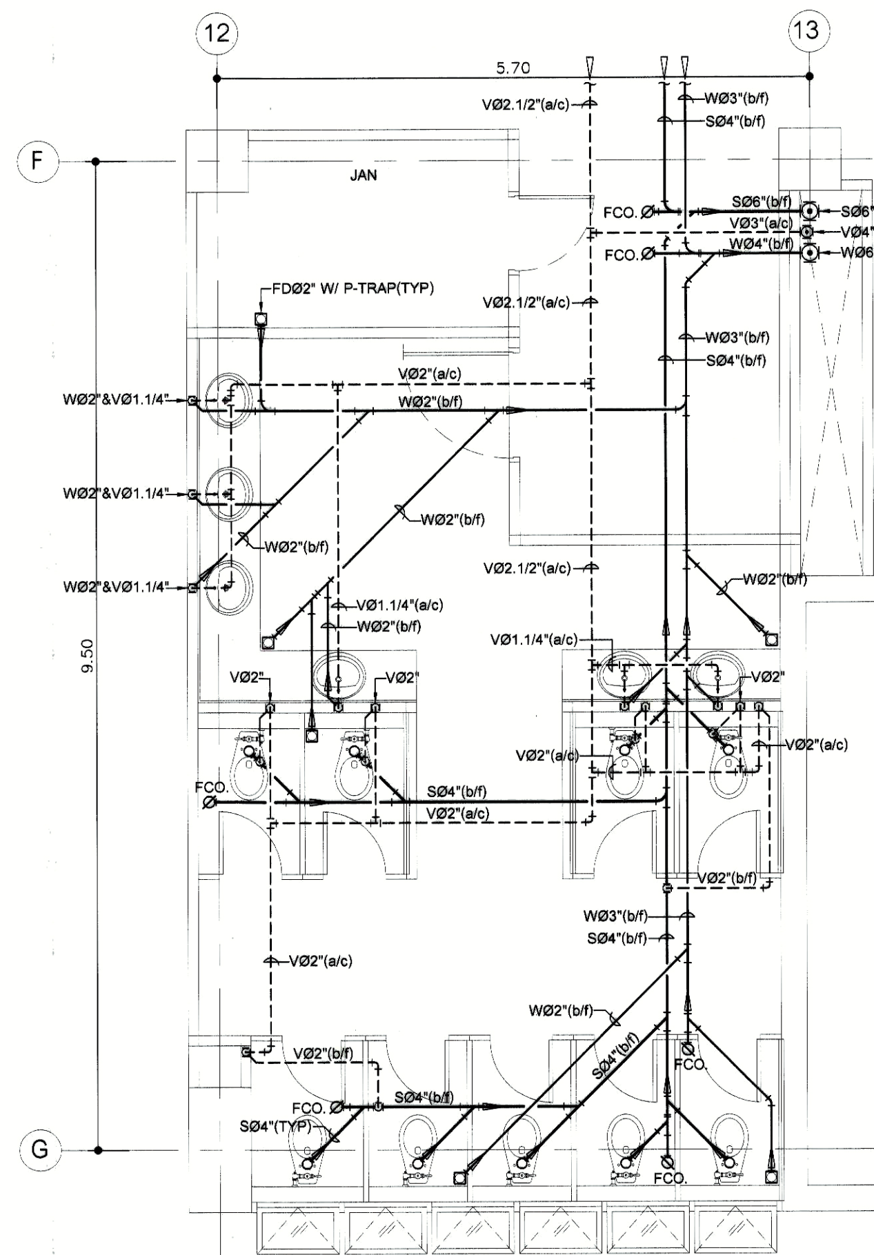
ห้องน้ำ T-501 (CW) มาตรฐาน 1:50
